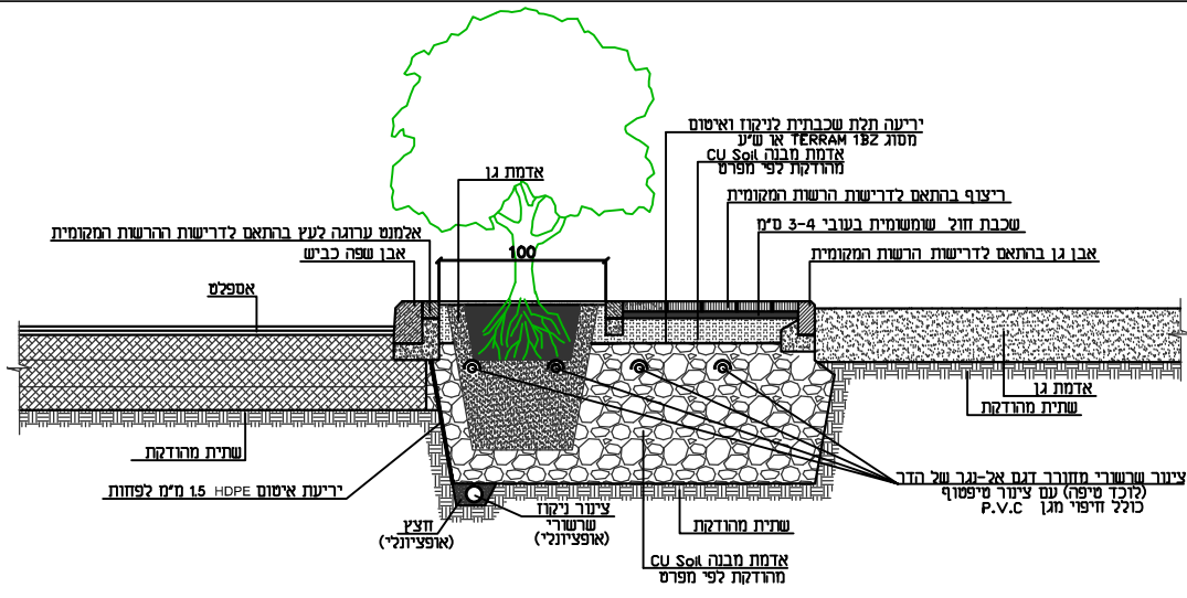
חתך ב-ב קנ"מ 1:50
