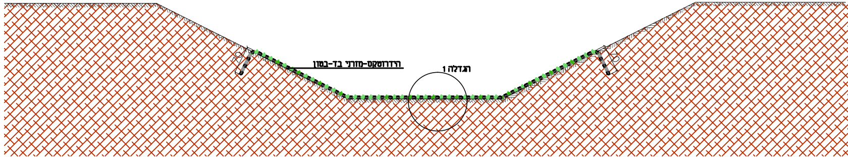
חזתך אופייני קנה מידה 1:100
