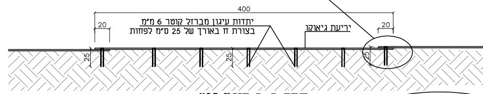
חתך ב-ב קני"מ 1:25
