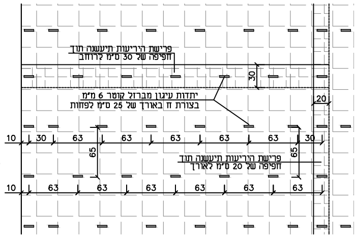
מערך יתדות עיגון
