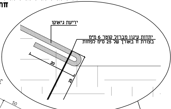
פרט קצה תחתון
